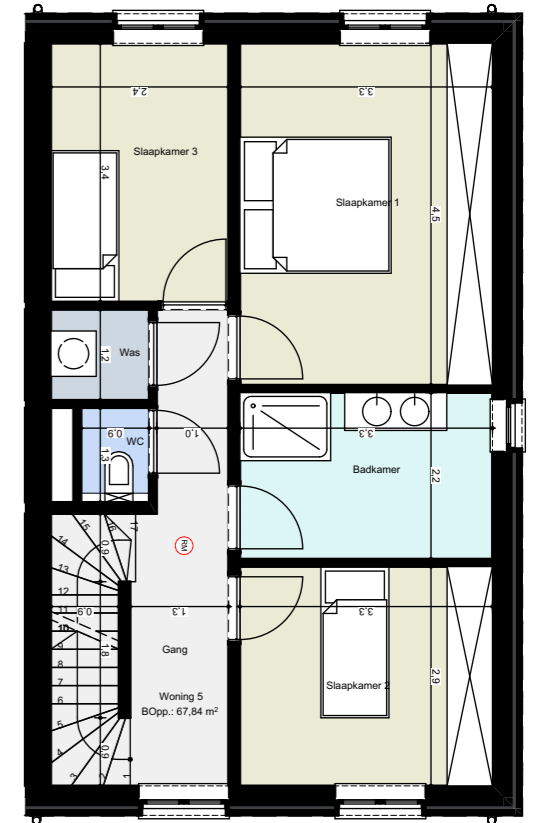
1ste verdieping:
