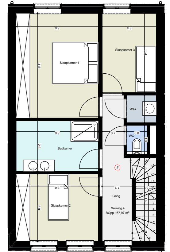
1ste verdieping:
